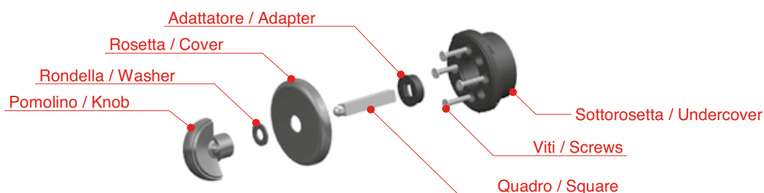
Maniglia girevole / girevole Handle / Handle
