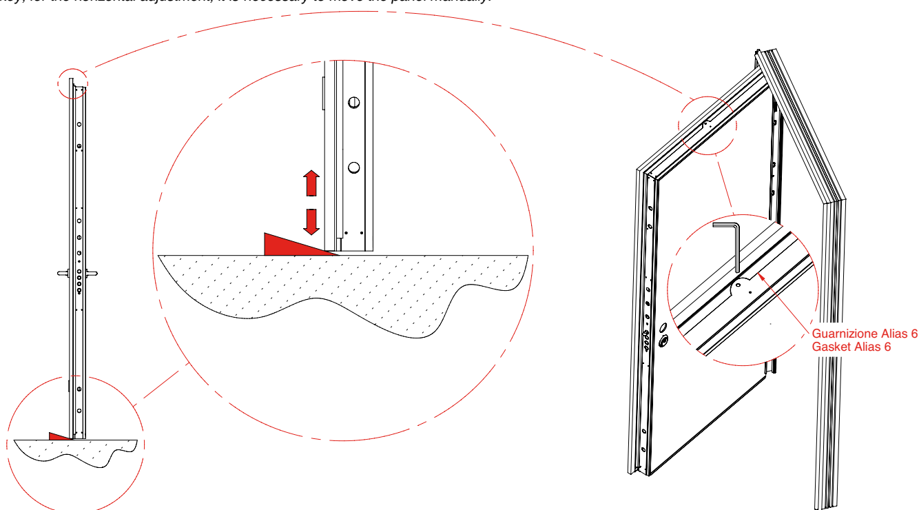
Vista pre-foratura carena con guarnizione Alias 6 rimossa
