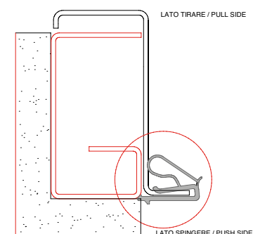
POSIZIONE GUARNIZIONE - Gasket position
