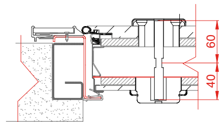
Soluzione per FLAT (Sp. pannello interno 10-15mm) Flat solution (10-15mm thickness internal panel)
