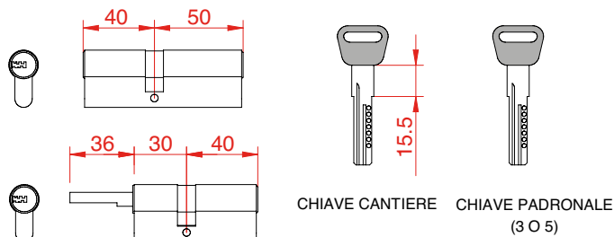
CILINDRO DI SICUREZZA / SAFETY CYLINDER
