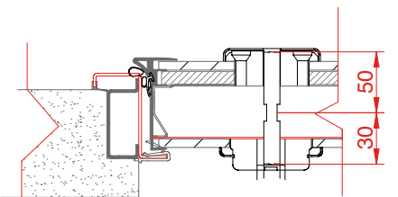
Soluzione per ZTL ZTL solution
