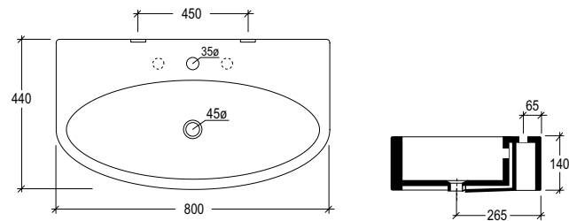
cod. BOLAVBW80 Lavabo Boing monoforo 80 appoggio, sospeso o su colonna (senza foro, tre fori su richiesta) Boing 80 one hole washbasin, countertop or wall-hung or on pedestal (without hole, three holes on request)
