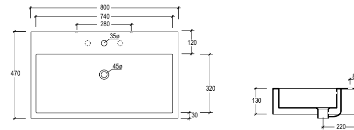
cod. QUALAV80 Lavabo Quad monoforo cm. 80 appoggio o sospeso (senza foro o tre fori su richiesta) Countertop or wall-hung washbasin Quad one hole cm 80 (without hole or three holes on request)
