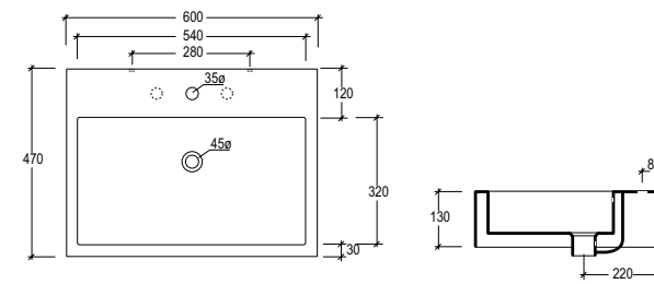
cod. QUALAV60 Lavabo Quad monoforo cm. 60 appoggio o sospeso (senza foro o tre fori su richiesta) Countertop or wall-hung washbasin Quad one hole cm 60 (without hole or three holes on request)
