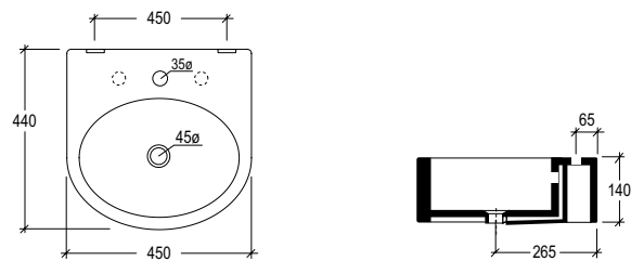
cod. BOLAVBW45 Lavabo Boing monoforo 45 appoggio, sospeso o su colonna (senza foro, tre fori su richiesta) Boing 45 one hole washbasin, countertop or wall-hung or on pedestal (without hole, three holes on request)
