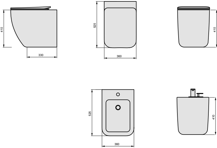
Wc Brio sospeso Wc Brio wall-hung Bidet Brio sospeso Bidet Brio wall-hung
