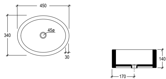
cod. BOLAVFS45 Lavabo Boing 45 appoggio, o su colonna Boing 45 washbasin countertop or on pedestal
